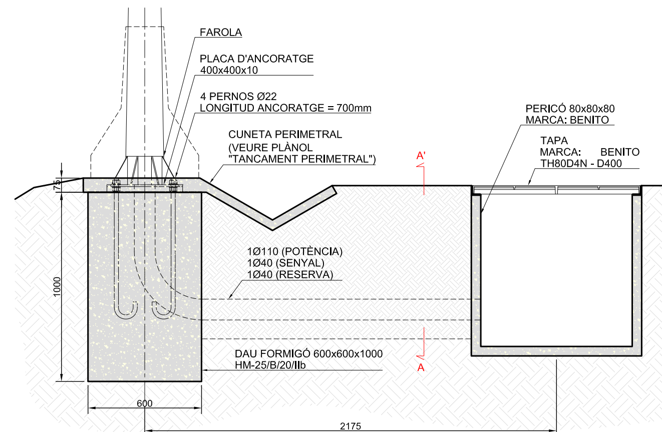
DETALL CONNEXIÓ FAROLA ESCALA 1:20
