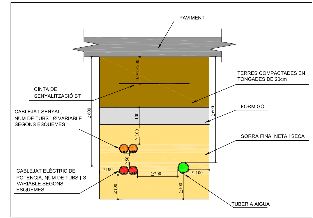
DETALL RASA AMB PROTECCIÓ DE FORMIGÓ
