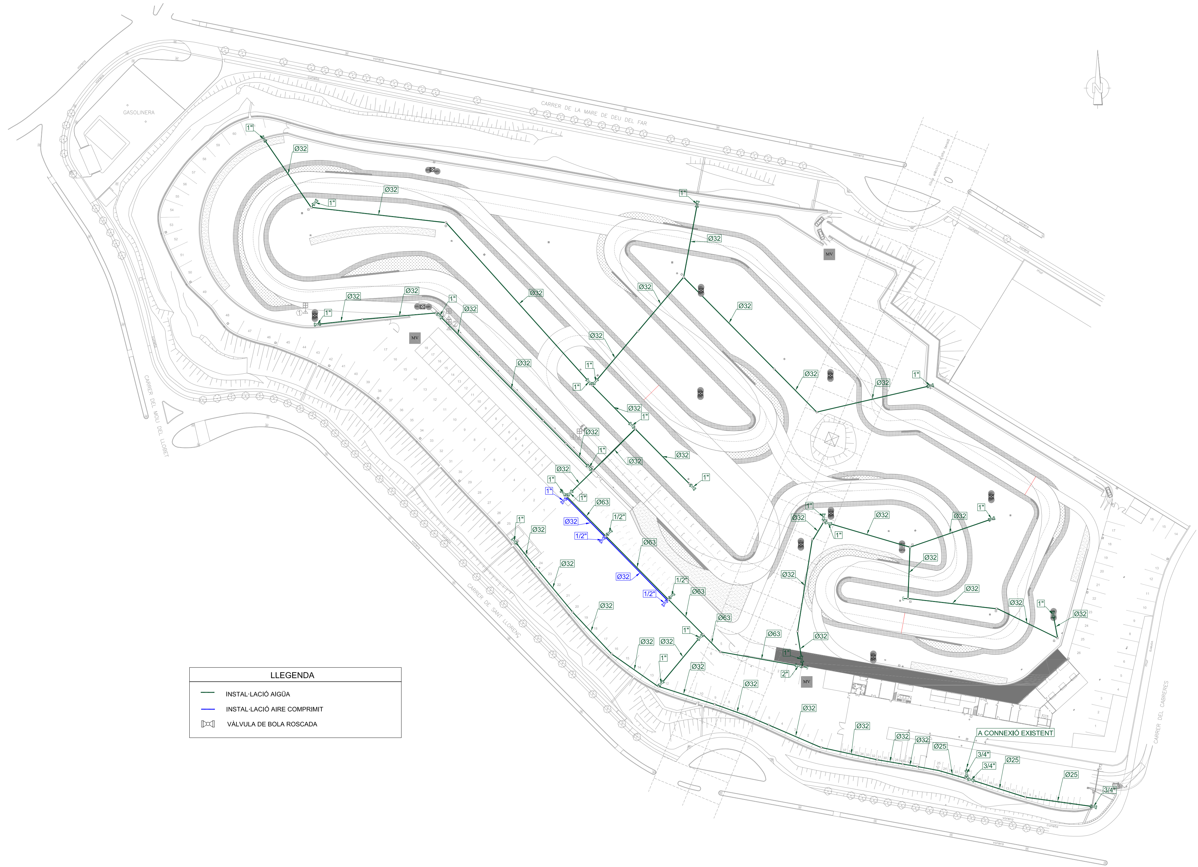
PLANTA E 1:1000
