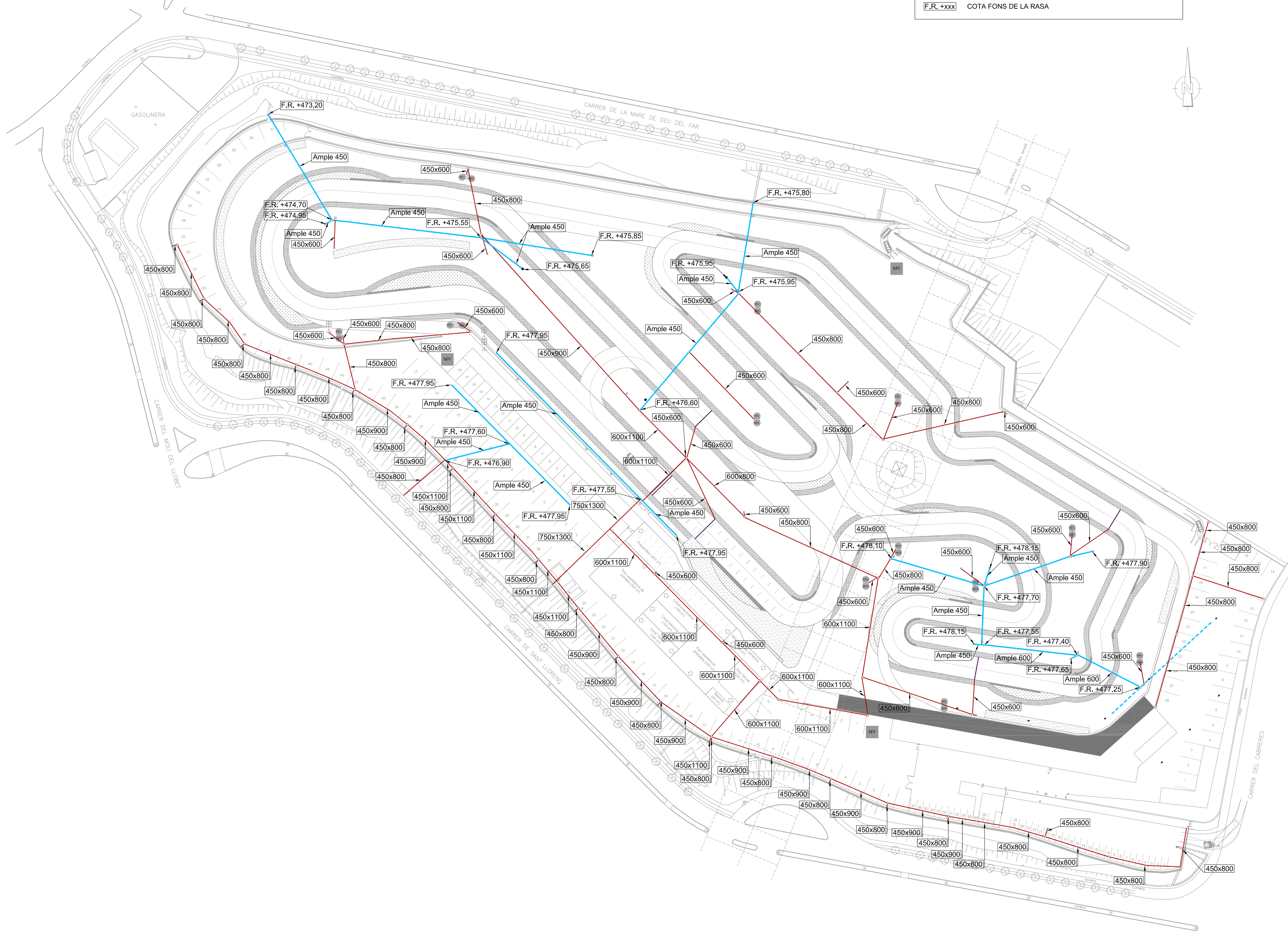
PLANTA E 1:1000
