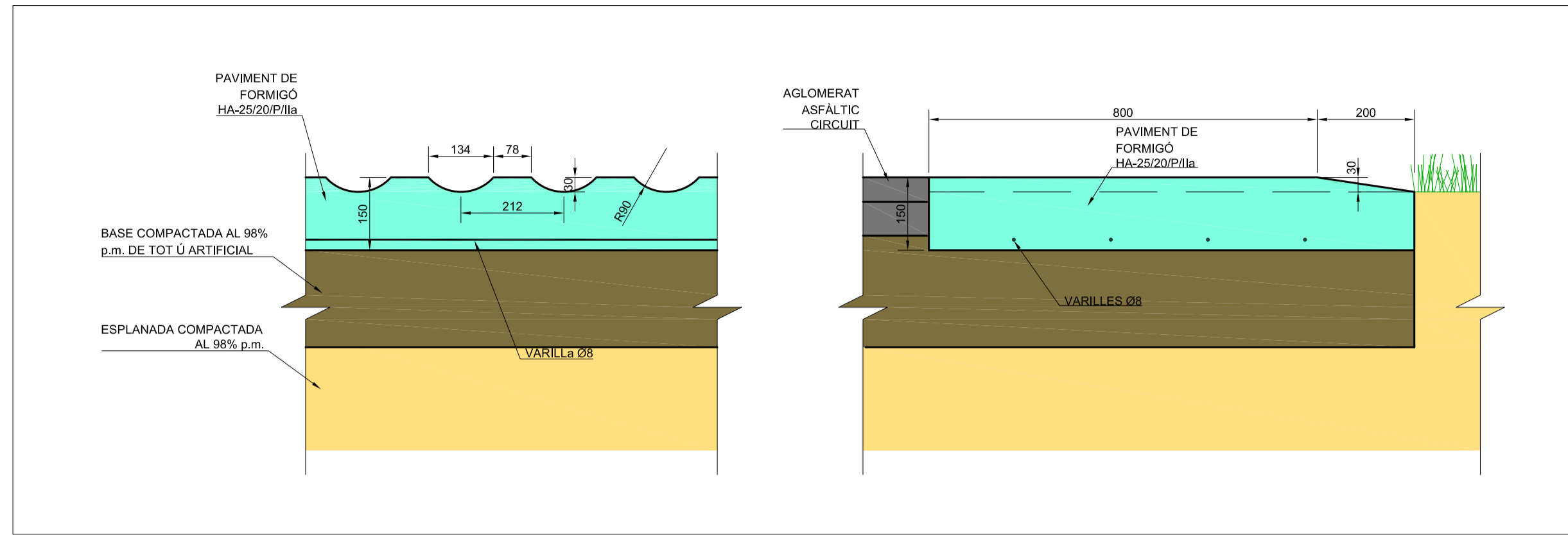
PIANO EXTERIOR - SECCIÓ LONG. E 1:10
