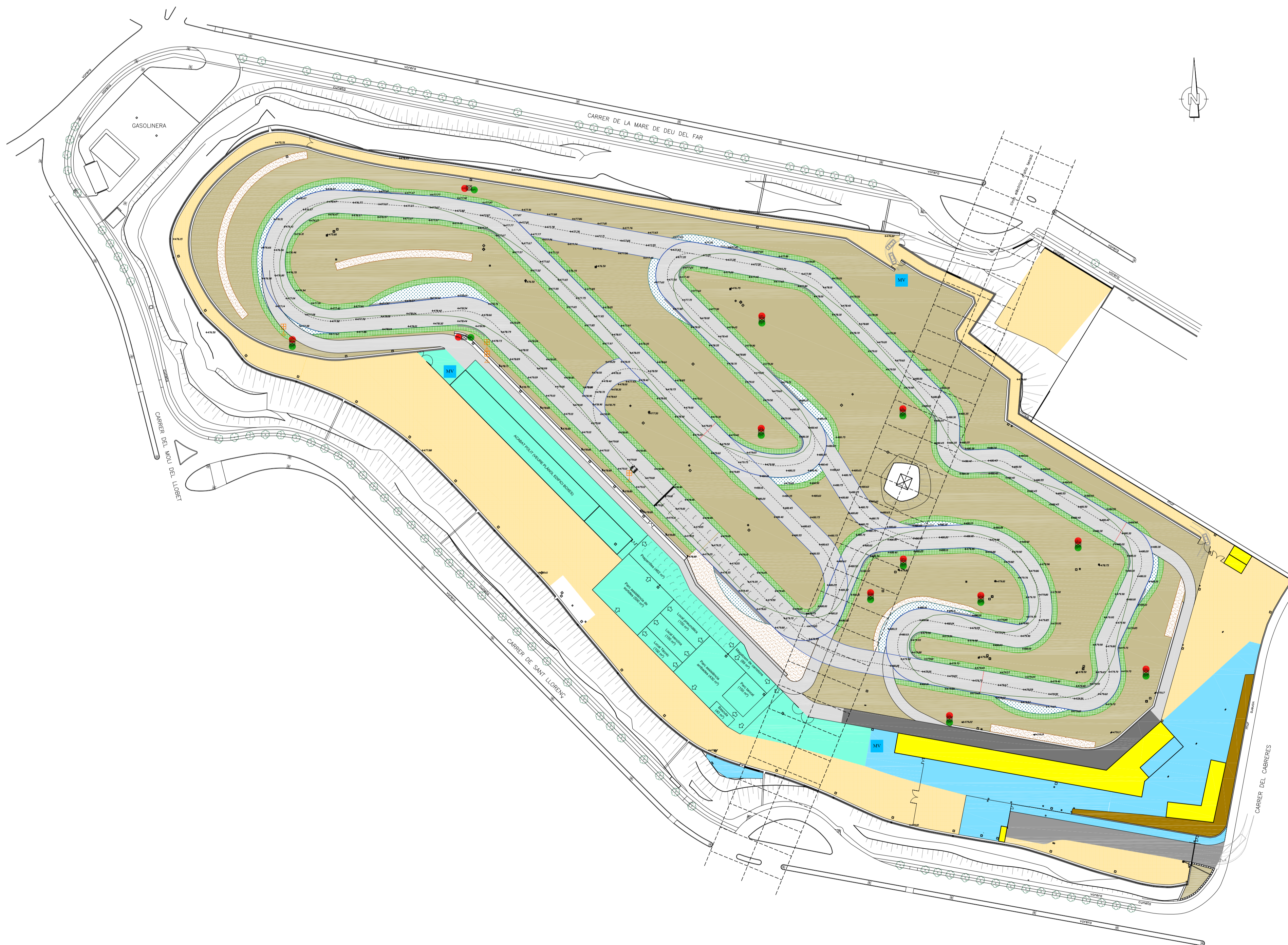
PLANTA DE PAVIMENTS E 1:1000
