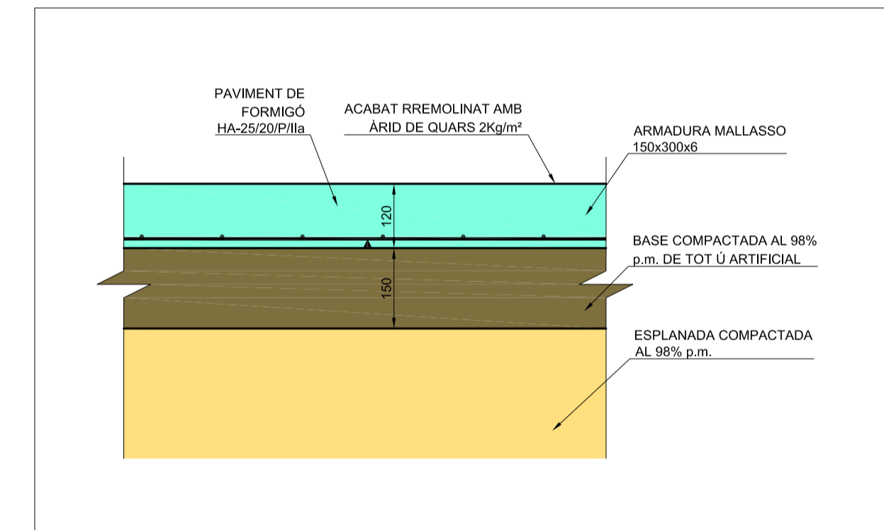
DETALL PAVIMENT FORMIGÓ E 1:10
