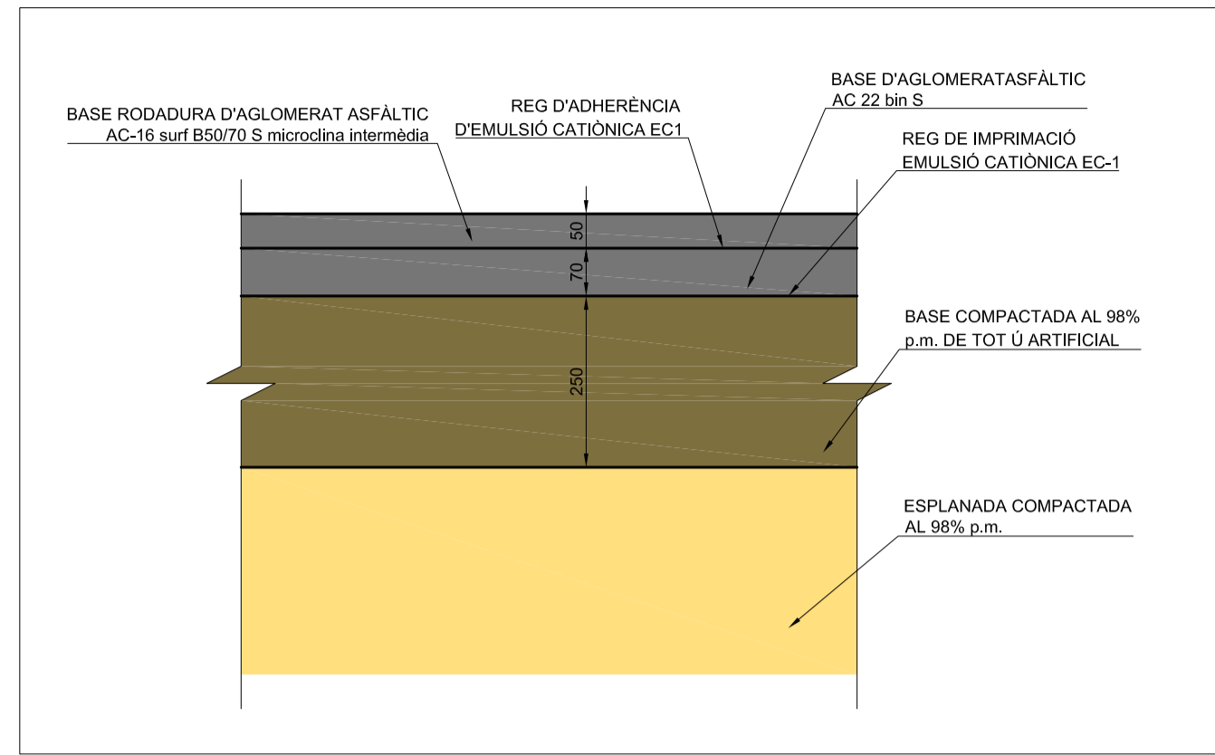
DETALL PAVIMENT D'AGLOMERAT ASFÀLTIC E 1:10
