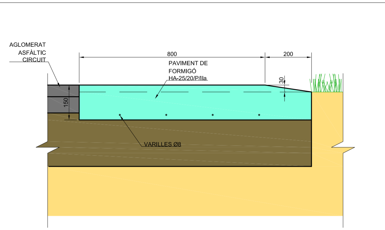
PIANO EXTERIOR - SECCIÓ TRANSVERSAL E 1:10
