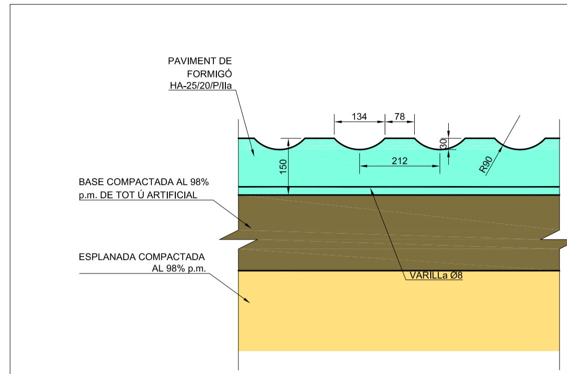
PIANO EXTERIOR - SECCIÓ LONG. E 1:10
